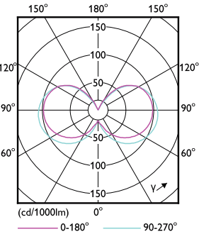
LEDbulb 75W E12 BA11 927 CL
