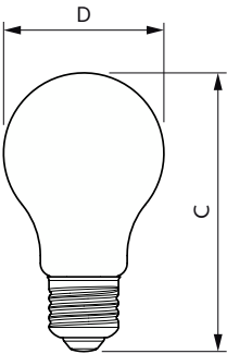
9.5A19/LED/950/FR/Glass/E26/DIM 1FB T20
