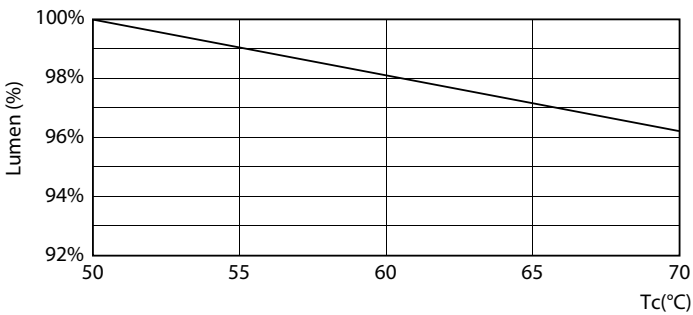
LEDtube COR 8,5W 50K LumenVsTc
